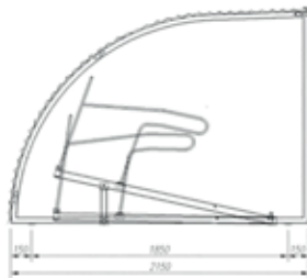
Vue latérale
